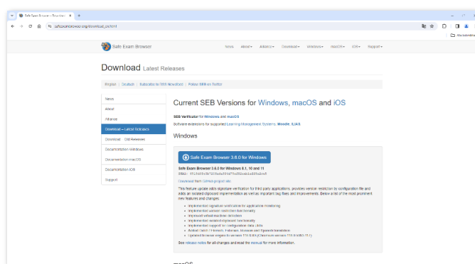
Bild 1. SEB:s webbsida.
